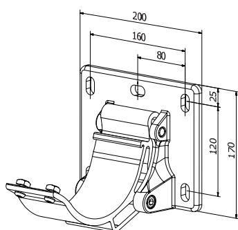
Monteringsbeslag til væg
