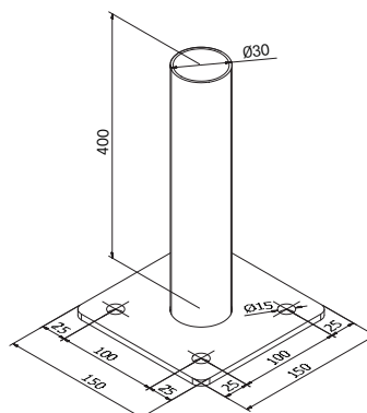
Monteringsplade for støtteben
