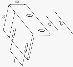
Vinkelbeslag for nichenmontering
