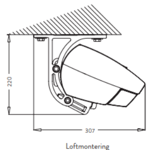
Loftmontering
