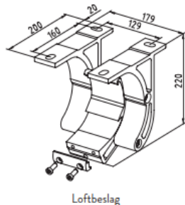
Loftbeslag
