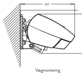
Vægmontering
