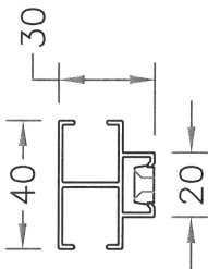
Dobbeltstyr
