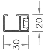
Enkeltstyr
